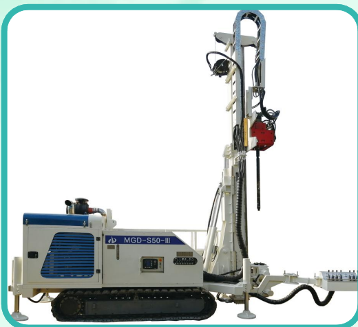
50米声频环保钻机
